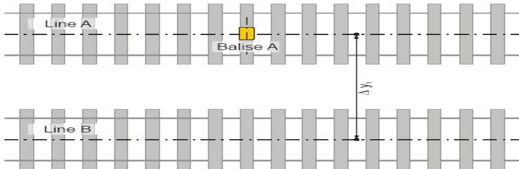
그림 25. 발리스의 병렬선로까지의 거리
