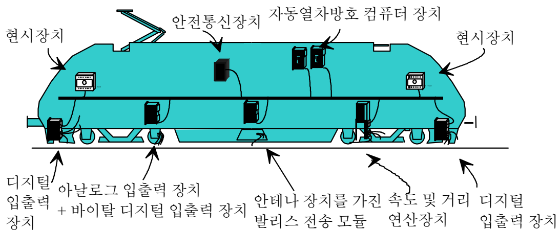
그림 9. 차내시스템의 분산설치(예)
