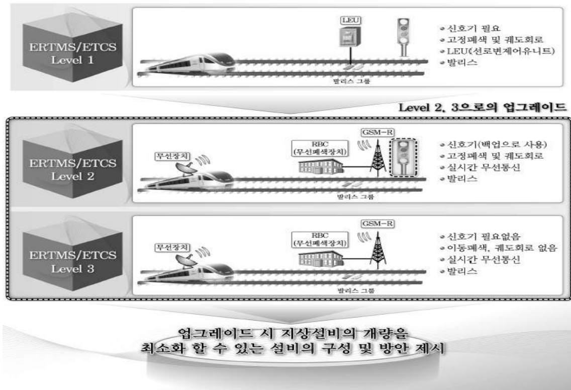
그림 1. ERTMS/ETCS 구성도
