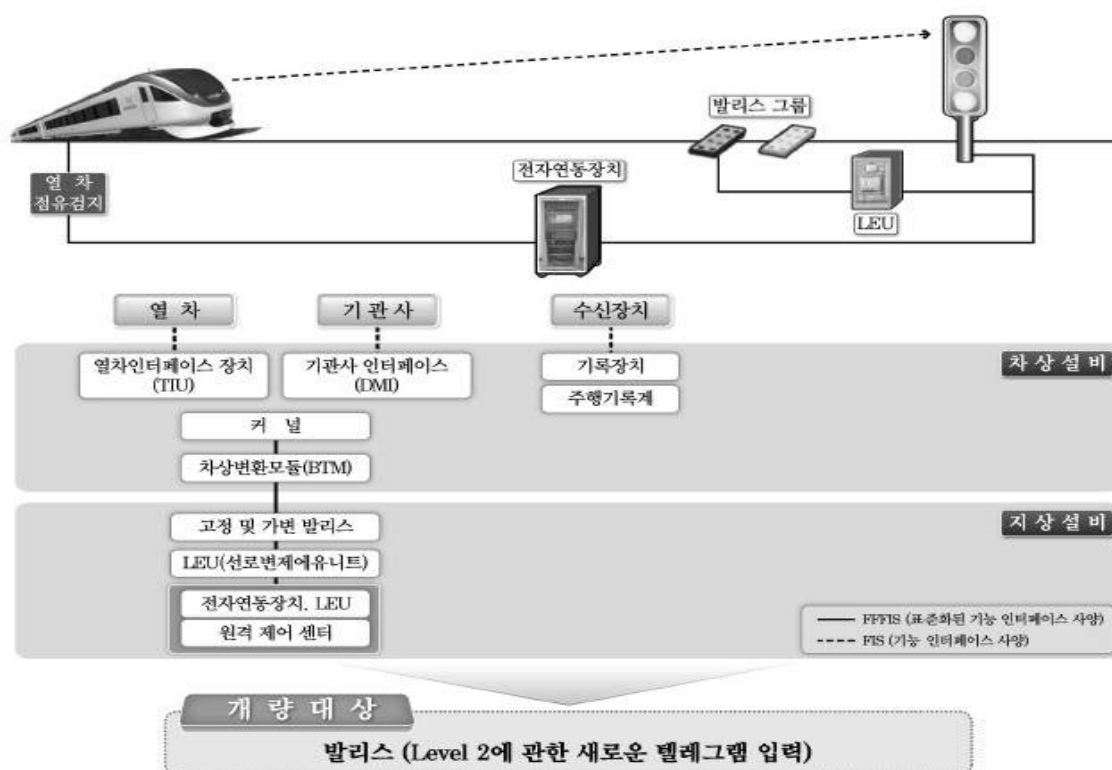
그림 2. ERTMS/ETCS Level 1 구성도
