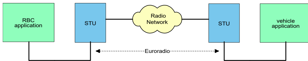
그림 14. 무선폐색센터와 열차 간의 인터페이스
