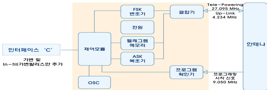
그림 21. 발리스 내부 구성도
