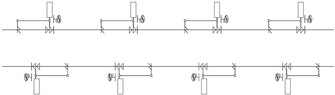
그림 19. 폐색구간(현장) LEU 구성
