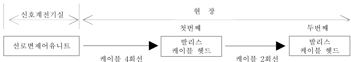
그림 14. 선로변제어유니트와 발리스 단자함간 케이블 설치도
