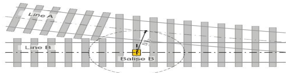
그림 26. 분기기 내의 발리스와 안테나의 최소거리
