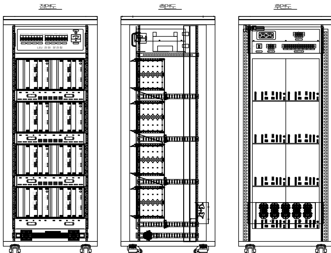
그림 18. 선로변제어유닛(실내용)(신호계전기실) 구성(LEU 서브랙 8개 기준)
