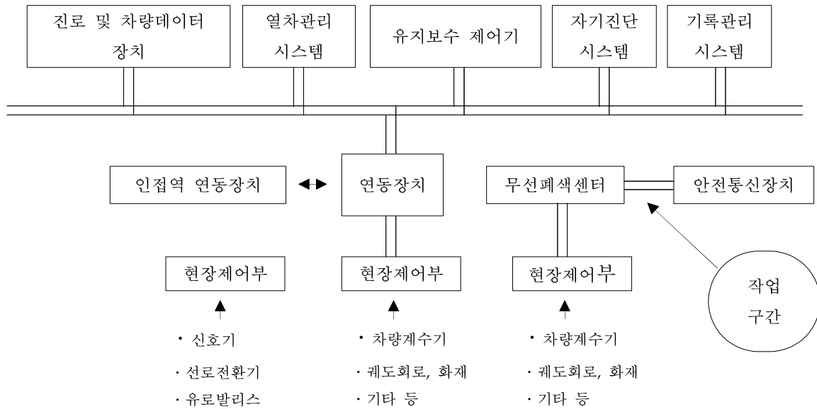
그림 8. ERTMS/ETCS 지상설비 구성
