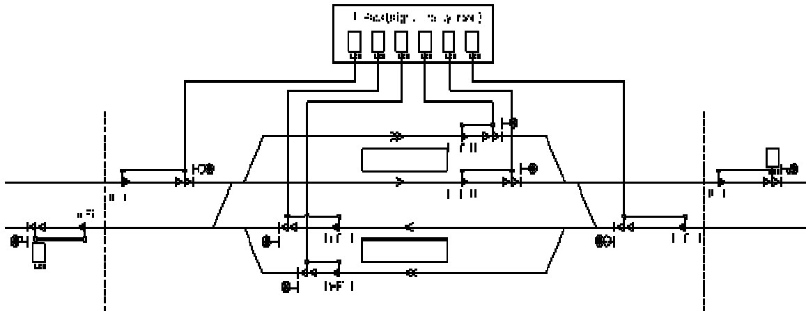
그림 17. 신호계전기실 LEU 구성
