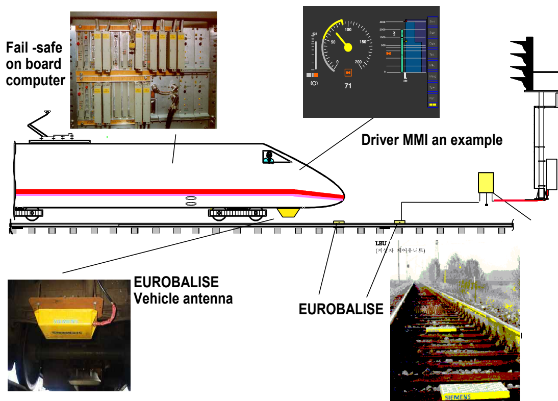
그림 7. 유럽열차제어시스템 구성
