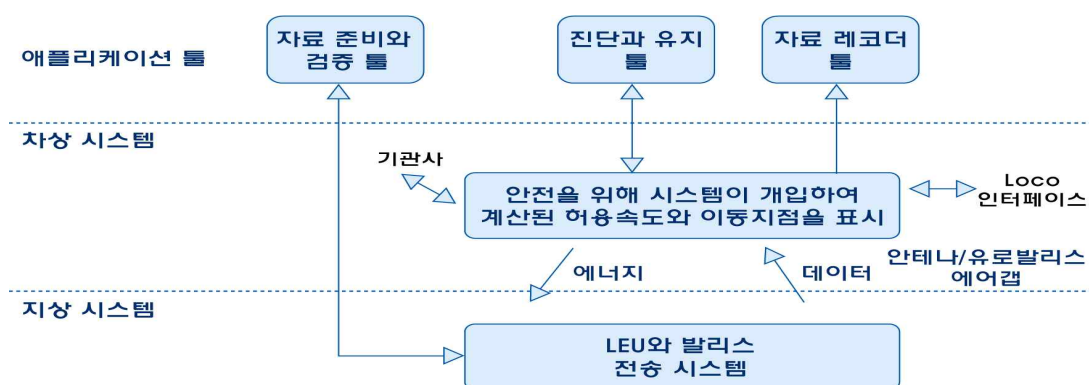
그림 15. ERTMS/ETCS시스템의 구조
