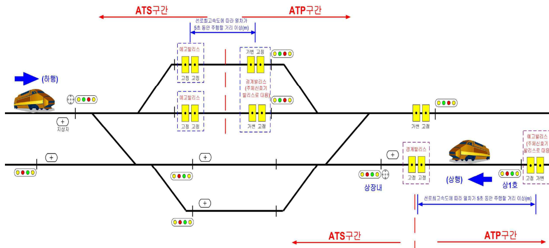
그림 8 ATS ↔ ATP운전모드 변경 구간의 일반적인 구성도
