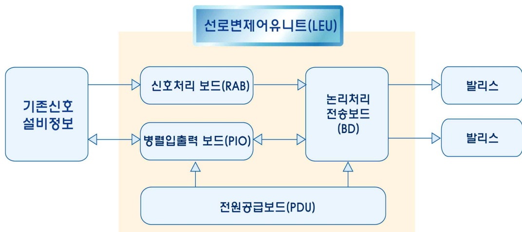
그림 20. LEU 구성도
