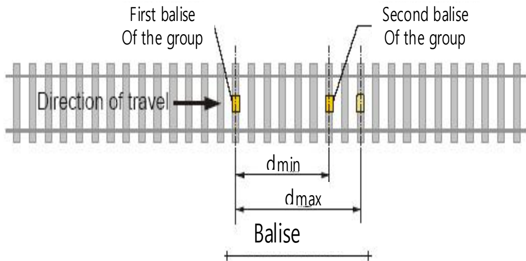
그림 24. 동일 발리스 그룹 내 발리스들 사이의 허용 간격
